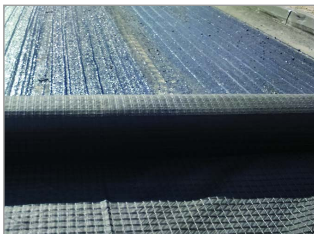
Укладка геосетки между слоями асфальтобетонного покрытия (препятствует образованию трещин в верхнем слое асфальтобетона)
