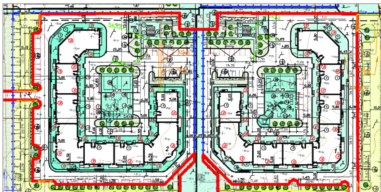
План благоустройства жилых домов № 1 и № 2 в мкр-не Тундровый
