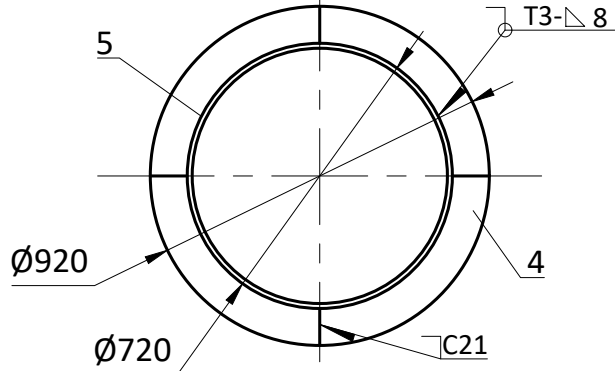
Б-Б (поз. 1, 2, 3 условно не показаны)
